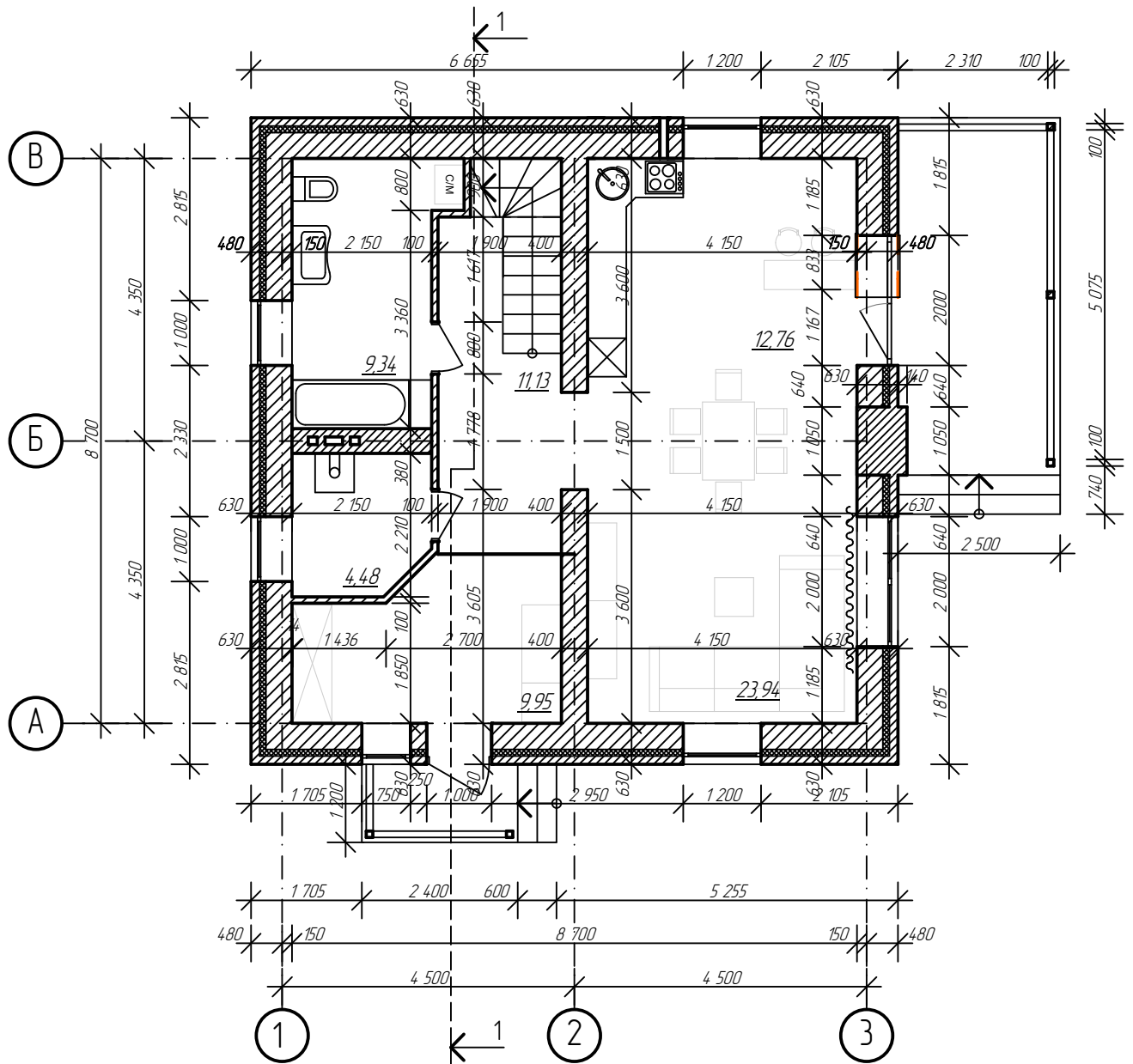
План 1-го этажа М 1:100
